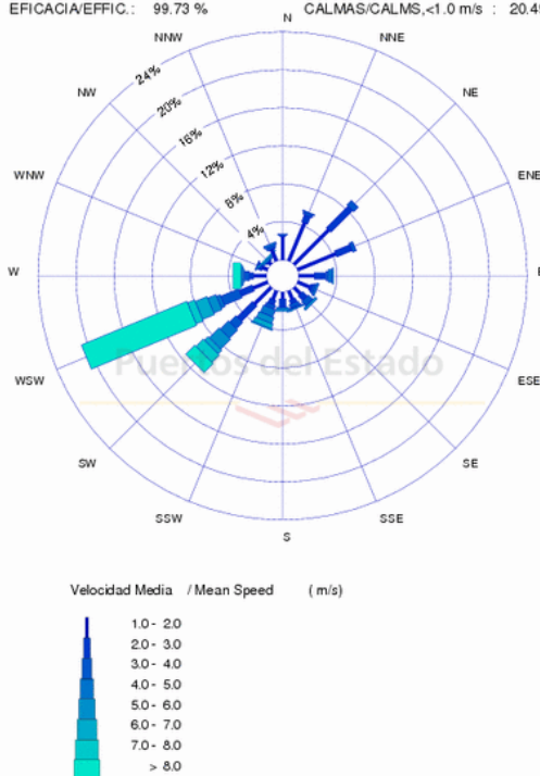
Figura 2. Rosa de los vientos correspondiente al mes de enero de 2016 (mareógrafo de Almería, fuente: Puertos del Estado).
