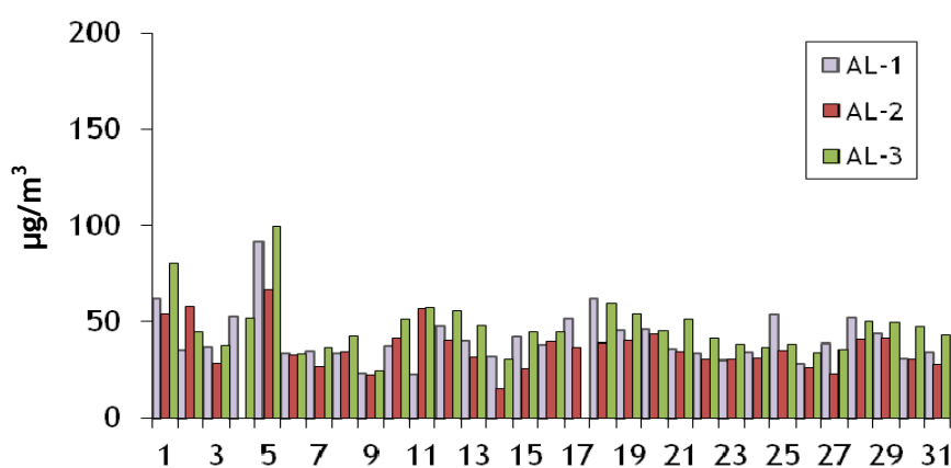
Figura 1. Evolución temporal de la concentración de partículas en suspensión en las estaciones de muestreo situadas en el Puerto de Almería. Agosto 2016.
