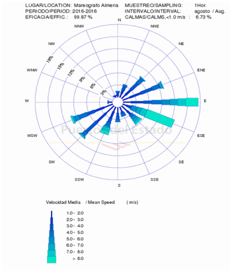
Figura 2. Rosa de los vientos correspondiente al mes de agosto de 2016 (mareógrafo de Almería, fuente: Puertos del Estado).
