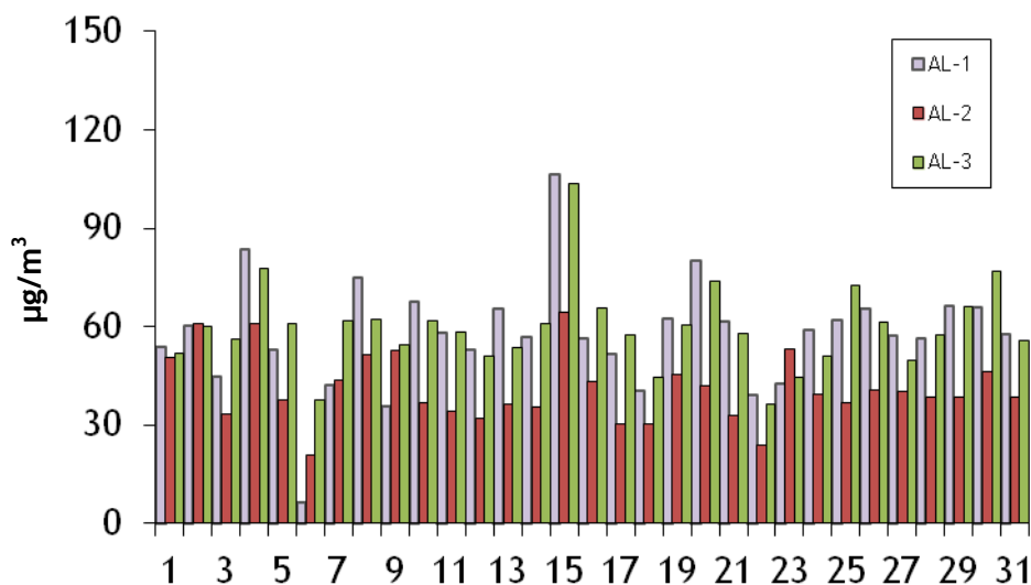
Figura 1. Evolución temporal de la concentración de partículas en suspensión en las estaciones de muestreo situadas en el Puerto de Almería. Julio 2018.
