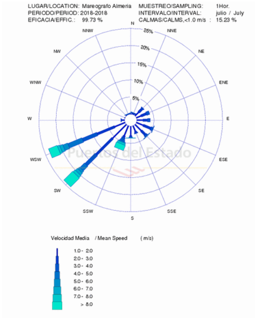
Figura 2. Rosa de los vientos correspondiente al mes de julio de 2018 (mareógrafo de Almería, fuente: Puertos del Estado).
